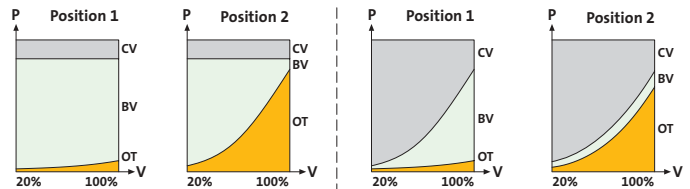
Druckabfall in einem System mit AB-QM
