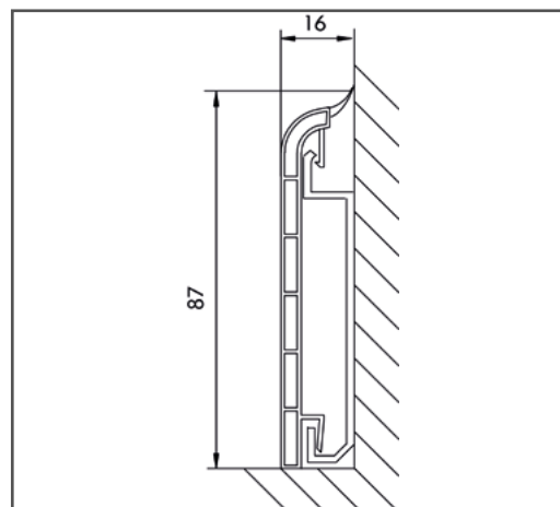
Abb. 2: Maßzeichnung HZ-Blindleiste BLF mit HZ-Blindleistenhalter BLH Artikel 155
