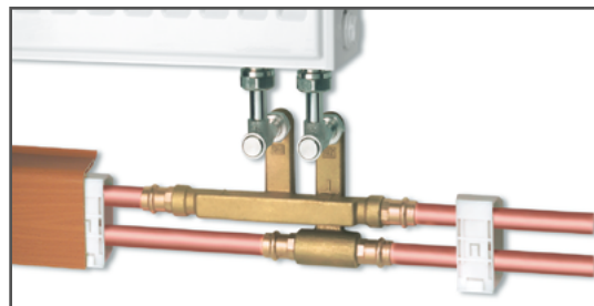
Abb. 8: HZ-Heizkörperanschluss
