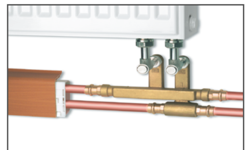
Abb. 5: HZ-Heizkörperanschluss
