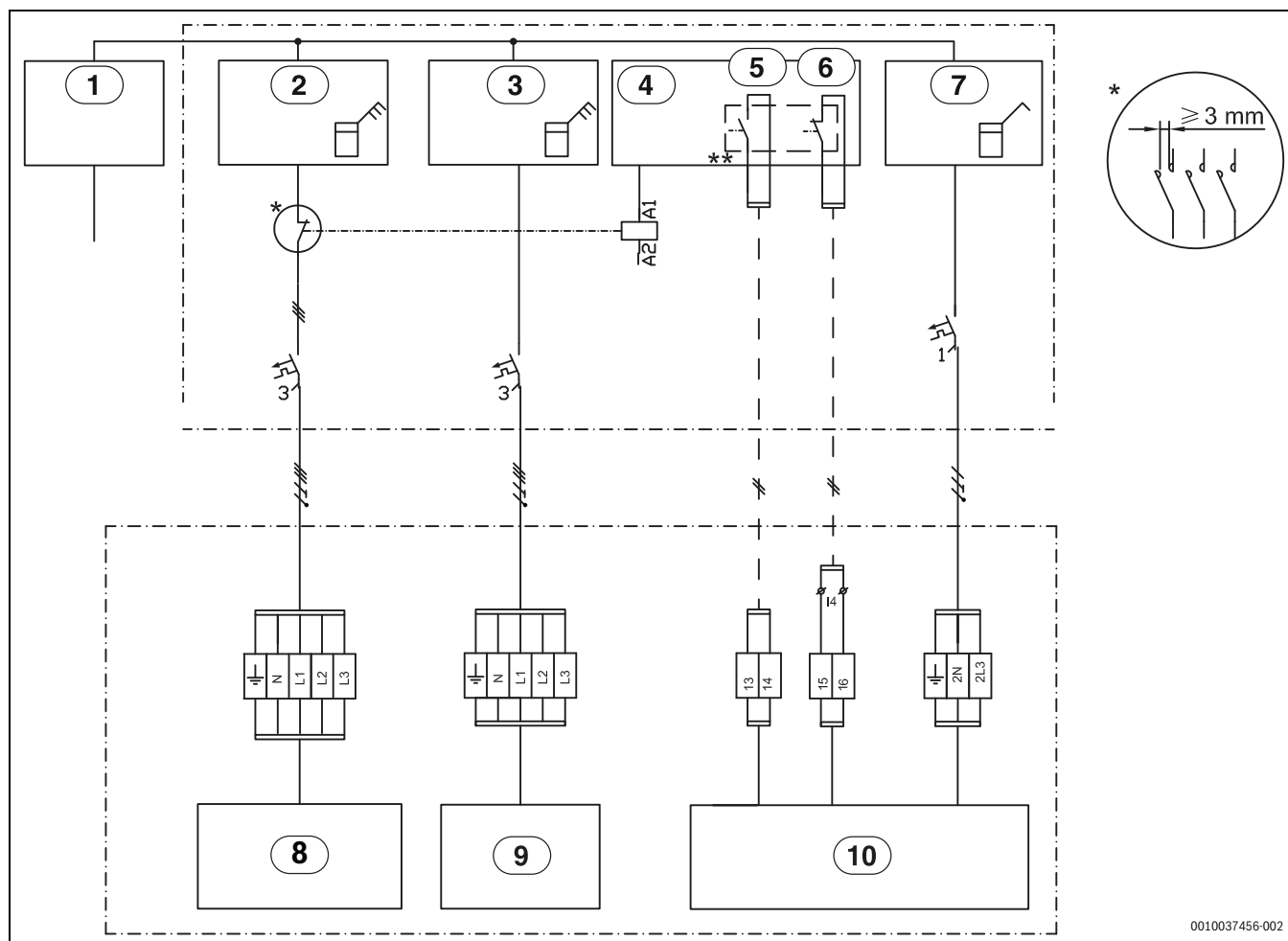
Bild 54 EVU Typ 2
