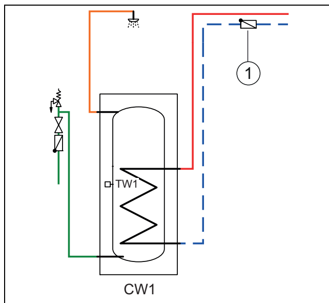
Bild 19 Warmwasserspeicher
