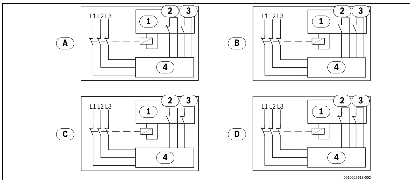
Bild 52 Anschlussplan für EVU/SG (3-phasig)
