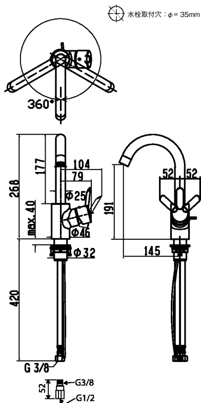
完成図
