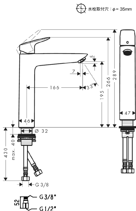
完成図
