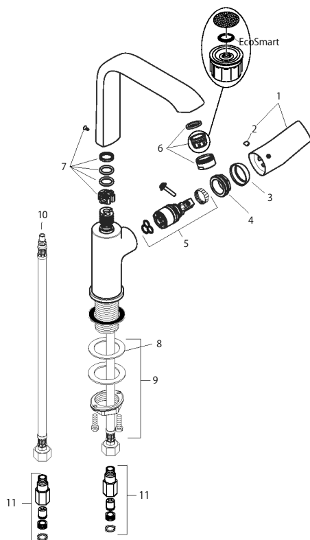
製品分解図
