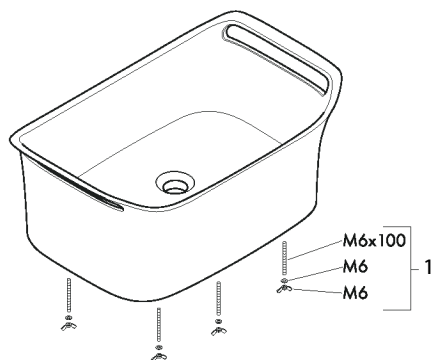
製品分解図
