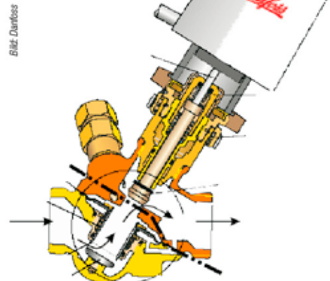
Bild 5 Das AB-QM-Kombiventil integriert einen Volumenstromregler und ein Regelventil. Die Differenzdruckregelung findet über dem gesamten Ventil statt, die Stellung des Regelkonus bestimmt den Durchfluss, der dann auch bei Druckschwankungen im Netz konstant bleibt.
