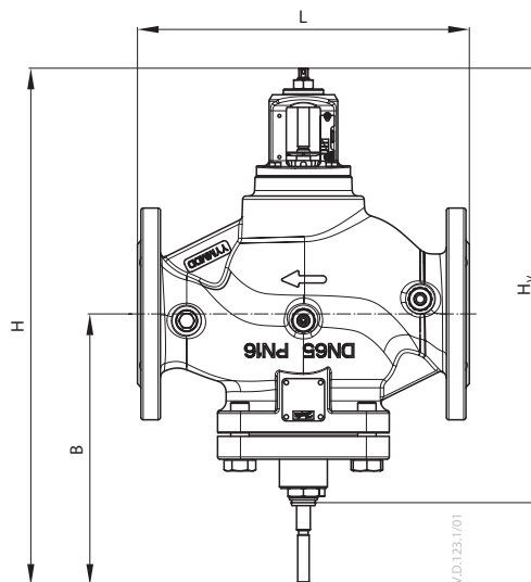
VFQ 22(1) DN 65-250
