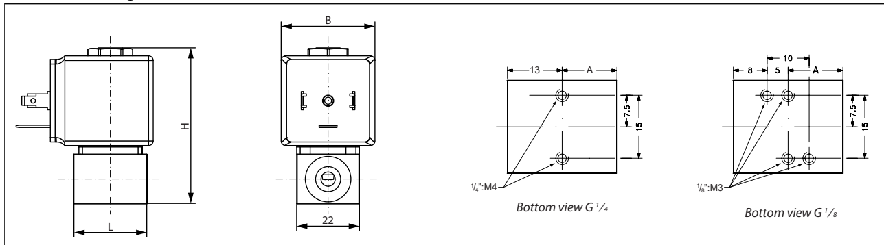
Bild 7: Abmessungen, Edelstahl
