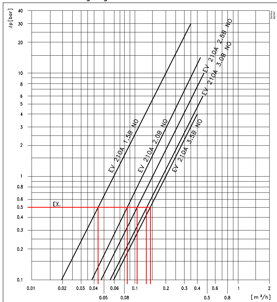
Bild 4: EV210A NO-Leistungsdigramm
