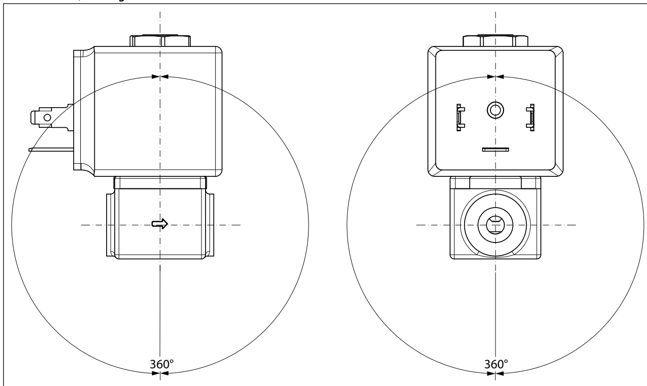
Bild 8: EV210A, Montagewinkel
