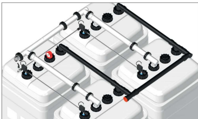
6. Fertig montierte Tankanlage.
