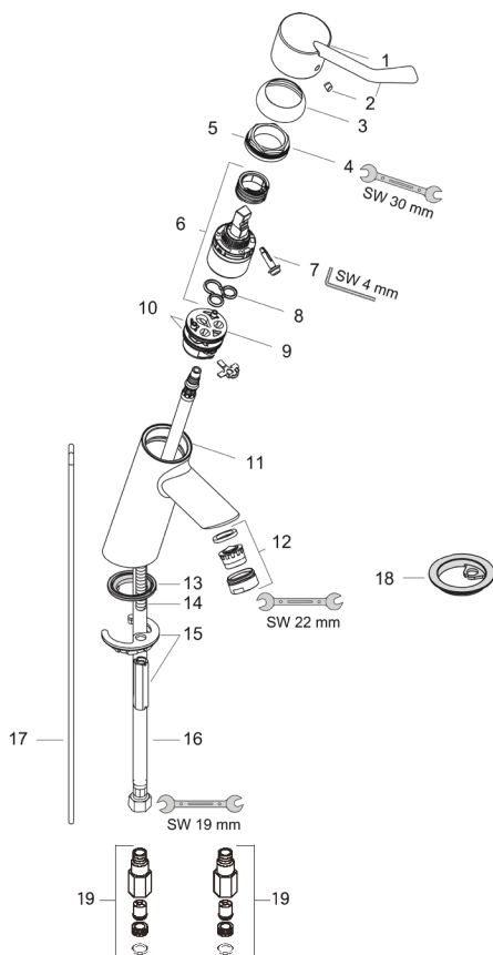
製品分解図
