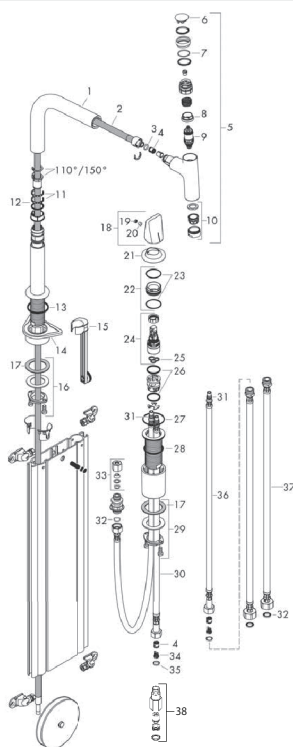
製品分解図
