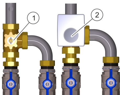
Abb. 20: Zwei-Zonen-Einschichtung
