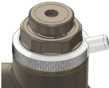
Abb. 38: Ventil aufdrehen
