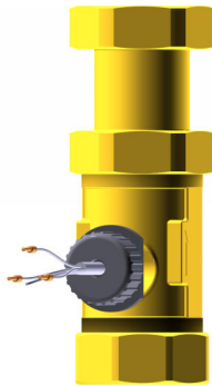
Abb. 14: Volumenstromsensor
