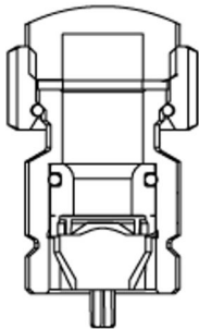
Abb. 12: Rückflussverhinderer
