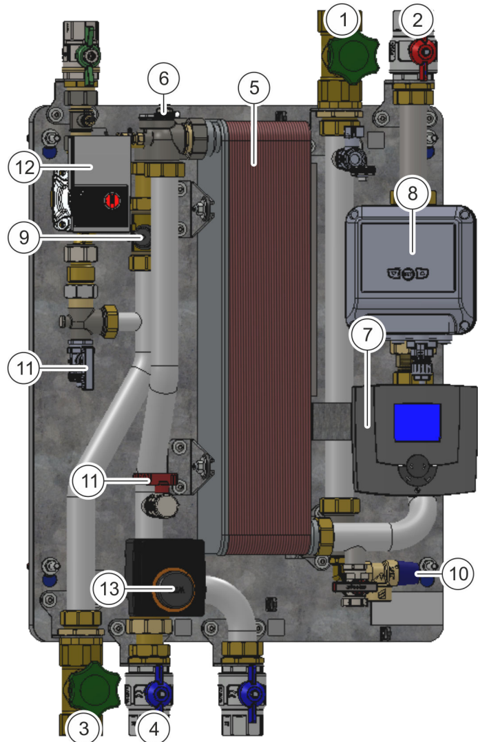
Abb. 1: Frischwarmwasserstation
