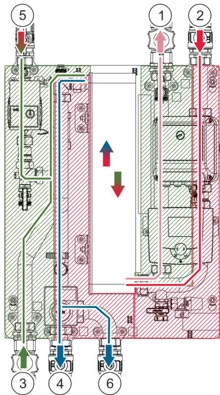
Abb. 6: Übersichtsschema der Leitungen
