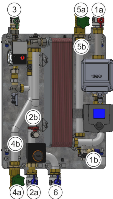
Abb. 27: Frischwarmwasserstation füllen
