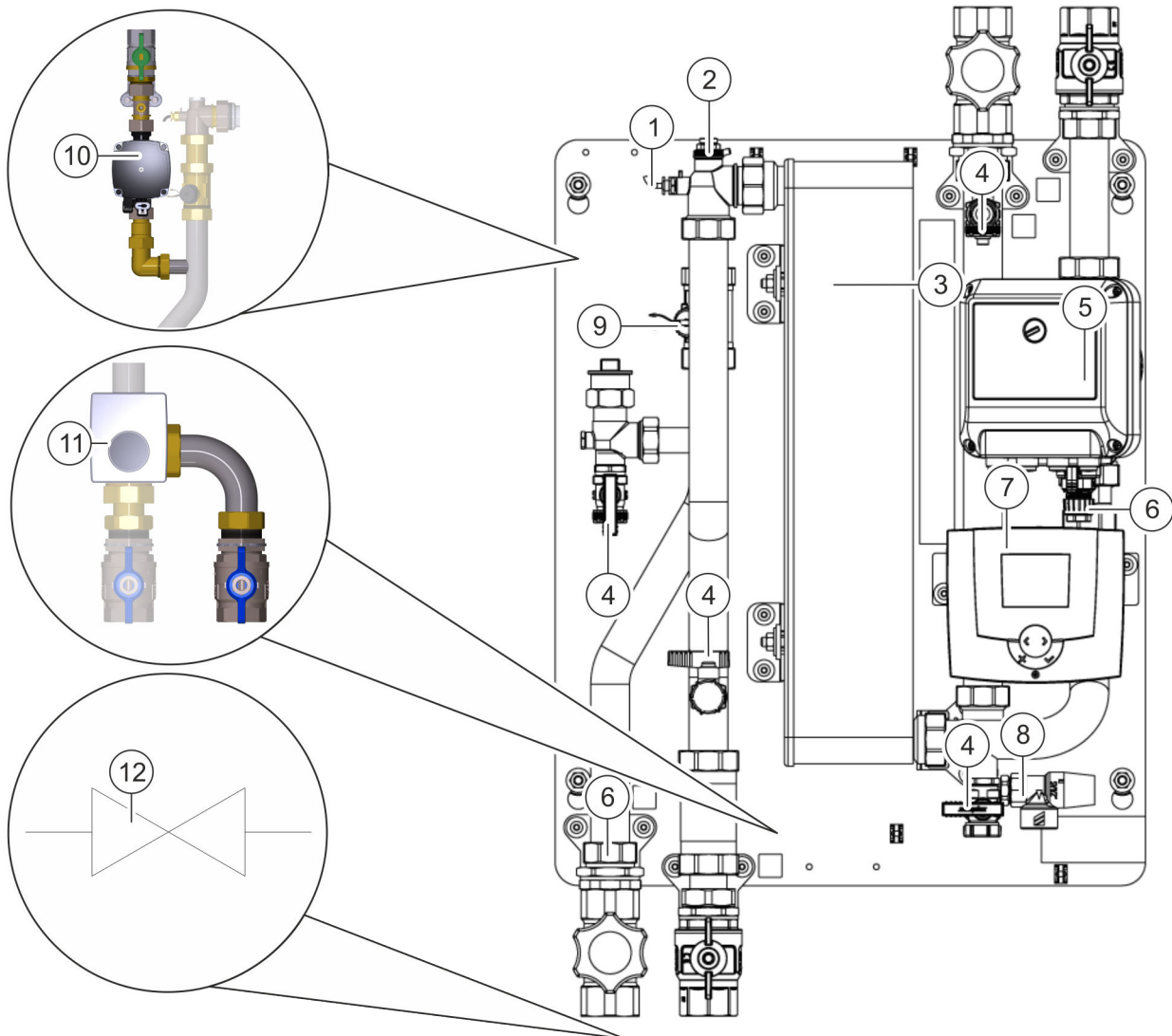
Abb. 7: Lage der Komponenten und Optionen
