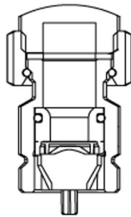
Abb. 5: Rückflussverhinderer
