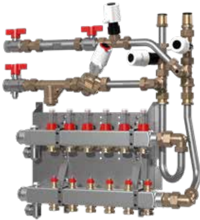
Abbildung: CDM-Modul Standard mit optionalen CSG-Verteiler, 6-fach
