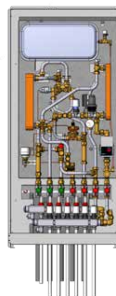
VX-F Station mit Verteilersystem
