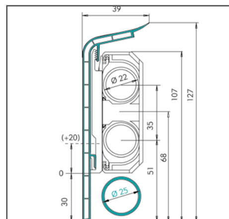
Abb. 3: Maßzeichnung HZ-SLL mit HZ-Schelle Artikel 2250 und drittem Rohr
