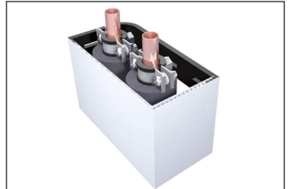
Abb. 9: HZ-Steigstrangprofil
