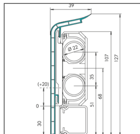
Abb. 2: Maßzeichnung HZ-SLL mit HZ-Schelle Artikel 2250 und zusätzlichem Kabelkanal
